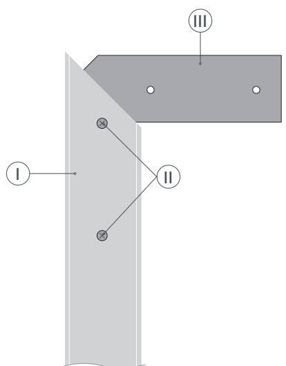
Вид сверху
