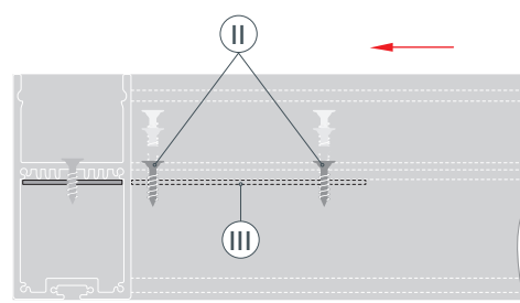
Вид сбоку
