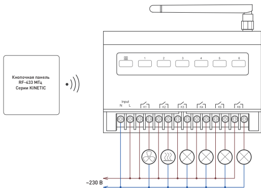
Рисунок 1. Пример схемы подключения релейного модуля TY-706-WF-SUF.
