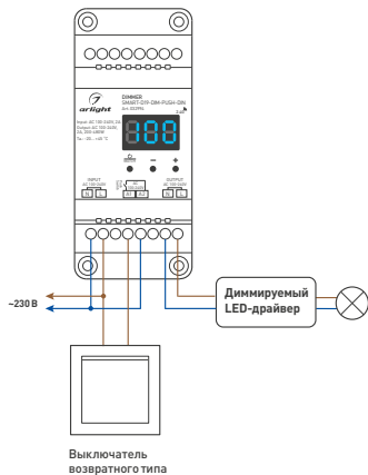
Рисунок 1. Схема подключения диммера SMART-D19-DIM-PUSH-DIN
